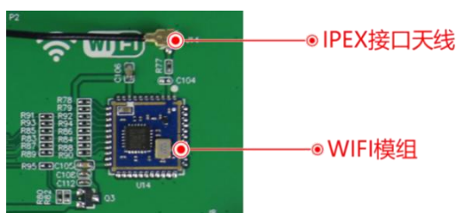
图 1-5 WIFI 配置图
