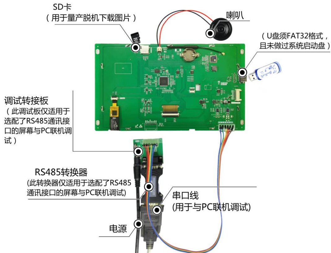
图 1- 6 调试工具
