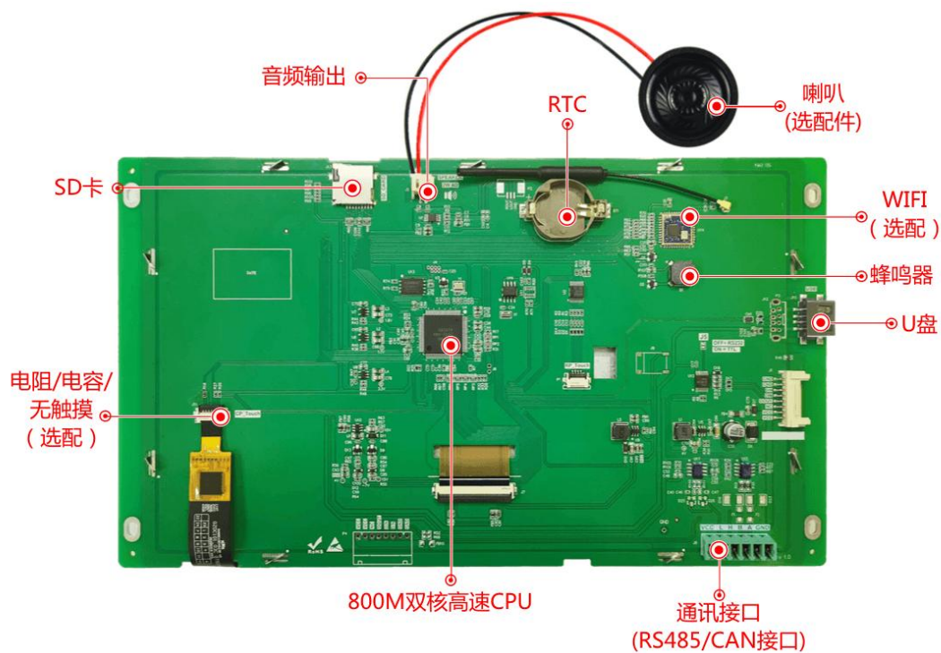
图 1-4 硬件配置图
